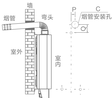
烟管背向安装 (图8)
