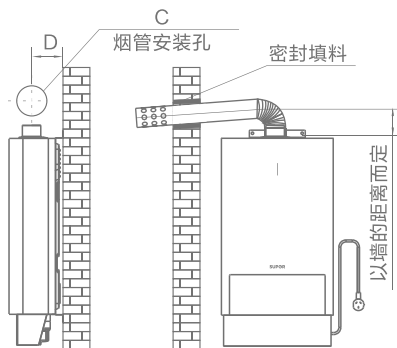
烟管侧向安装 (图9)
